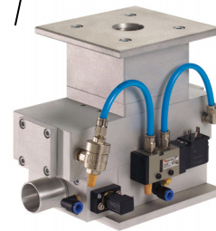
Metal Separator PROTECTOR
